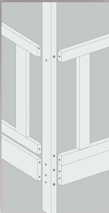
Узел сборки 1
