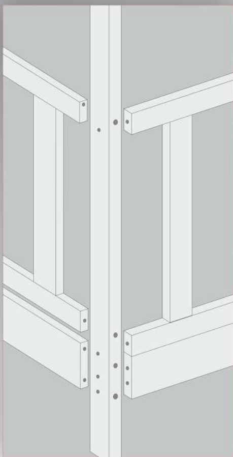
Узел сборки 3
