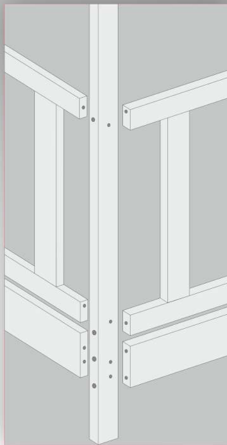
Узел сборки 4
