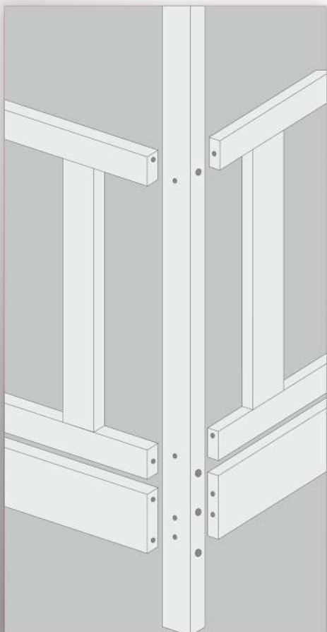
Узел сборки 3
